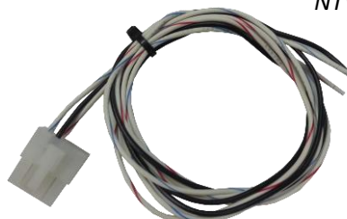
AVSW power/trigger harness NTV-HAR066
